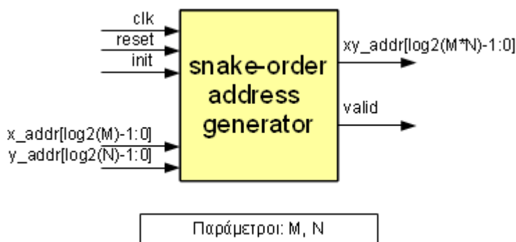
Σχήμα 1: Η διεπαφή της γεννήτριας διευθύνσεων snake-order.
