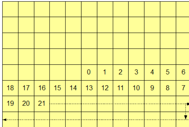
Σχήμα 2: Snake-order ακολουθία διευθύνσεων.
